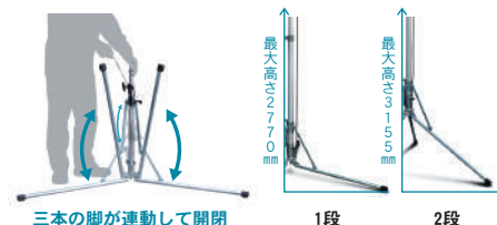
三本の脚が連動して開閉
